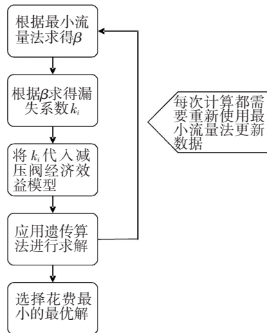
图1 减压阀经济效益模型求解流程
