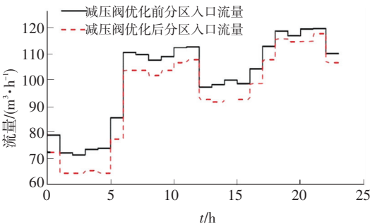
图 4 HJ 分区减压阀优化控制前后入口流量
